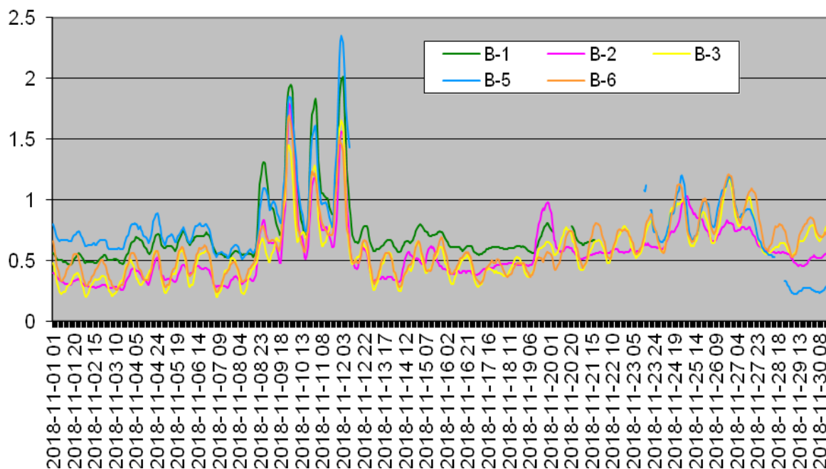
CO noiembrie 2018 Media mobila orara Valoare [mg/m 3 ]
