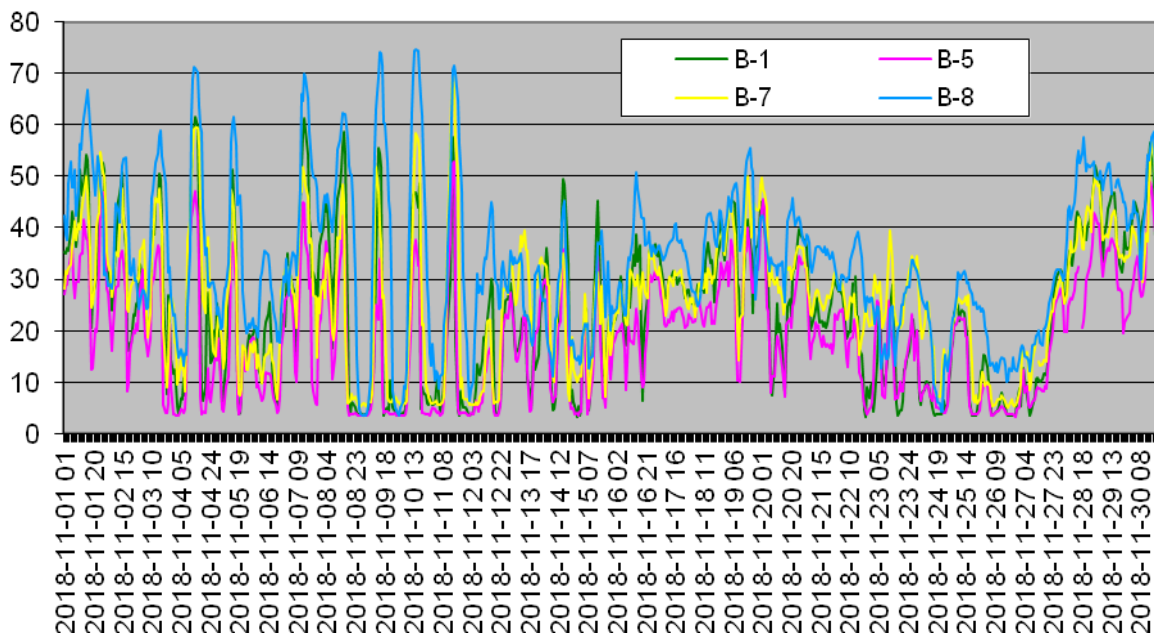
O3 noiembrie 2018 Valori orare Valoare [ \mu\text{g}/\text{m}^3 ]
