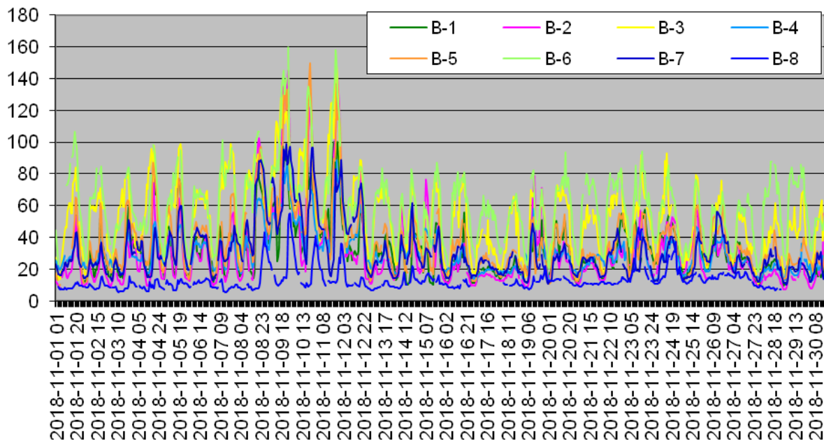
NO2 noiembrie 2018 Valori orare Valoare [ \mu\text{g}/\text{m}^3 ]
