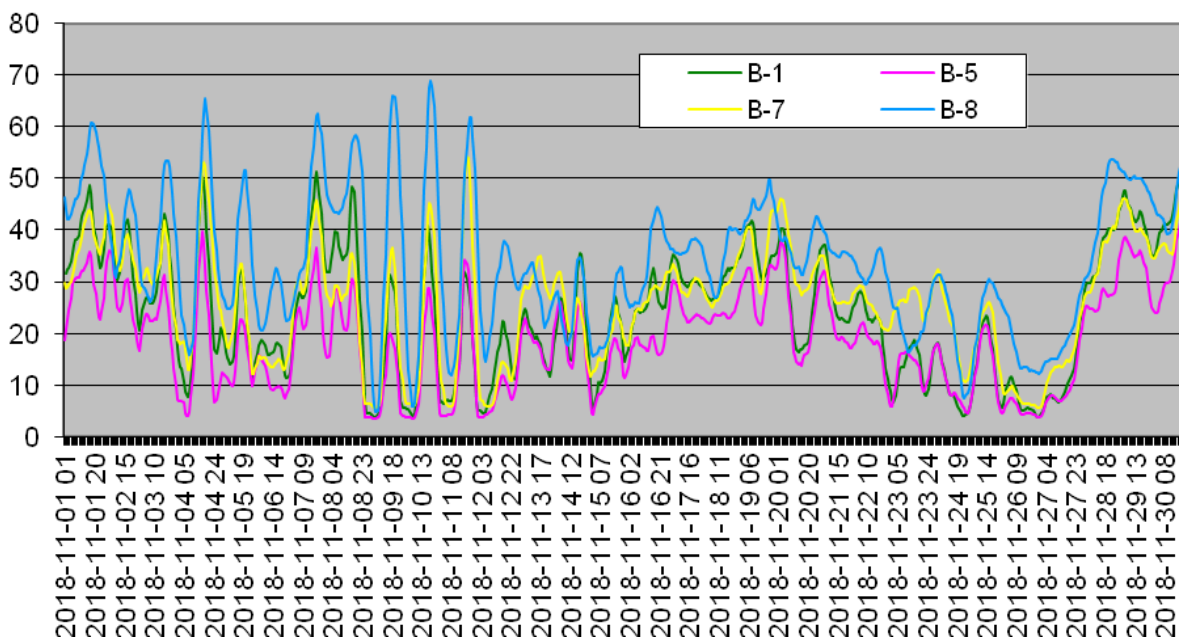
O3 noiembrie 2018 Media mobila orara Valoare [ \mu\text{g}/\text{m}^3 ]
