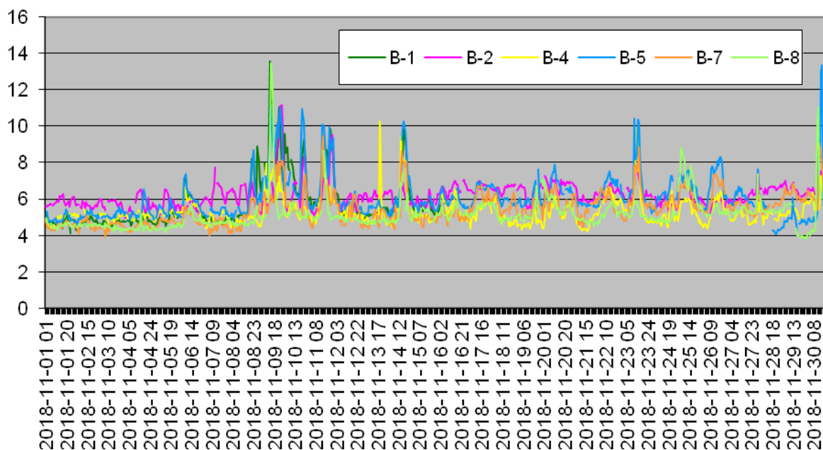
SO2 noiembrie 2018 Valori orare Valoare [ \mu\text{g}/\text{m}^3 ]
