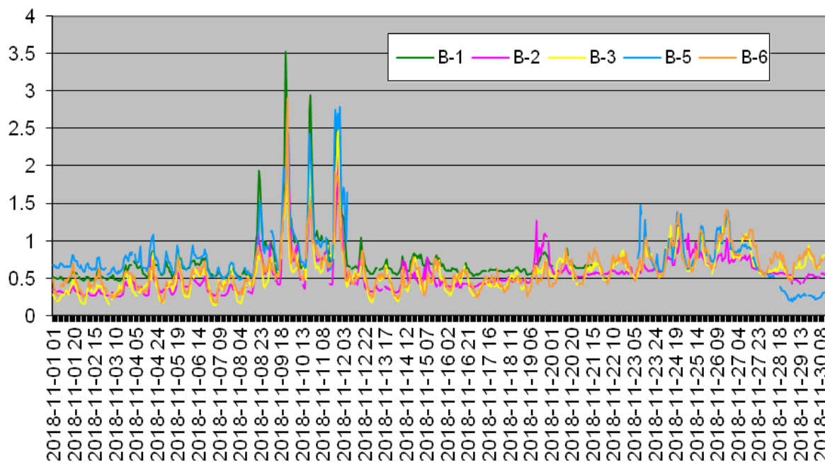
CO noiembrie 2018 Valori orare Valoare [mg/m 3 ]
